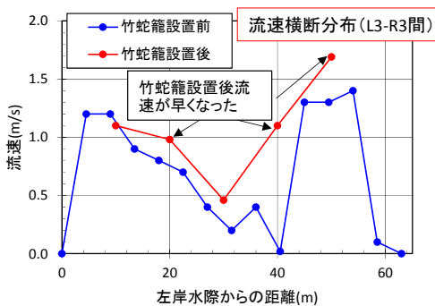
図-15 表面流速 (L3-R3間)
