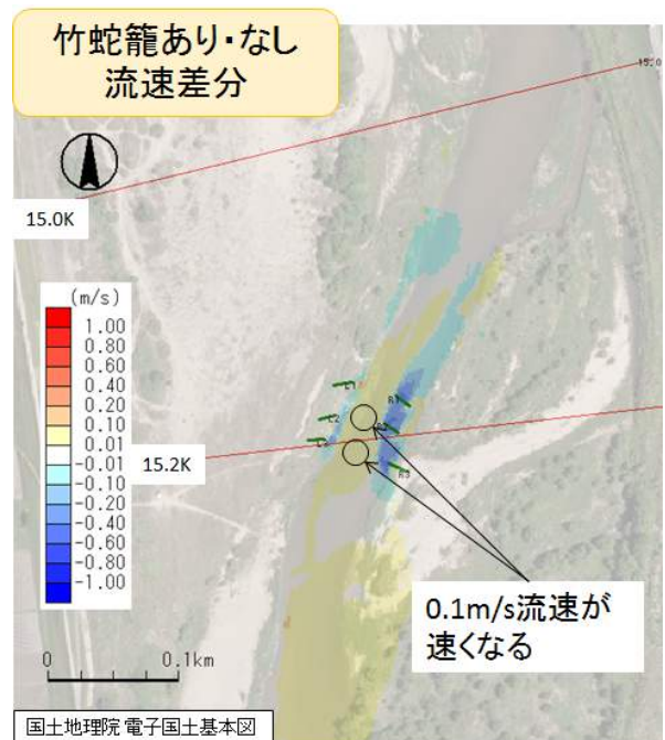
図-8 竹蛇籠あり・なしの流速差分
