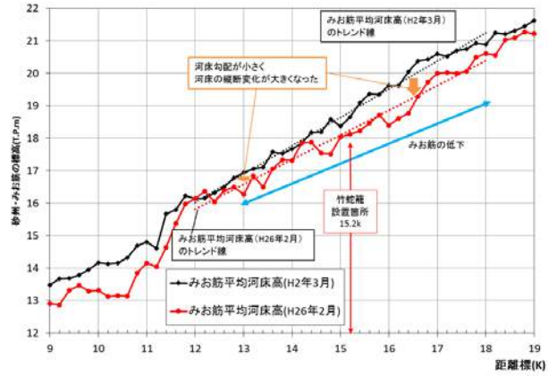
図-2 みお筋の河床高縦断面図
