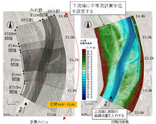
図-6 計算条件(左:メッシュ 右:河床高)
