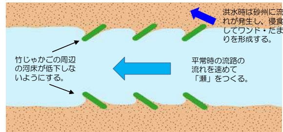
図-5 竹蛇籠効果のイメージ
