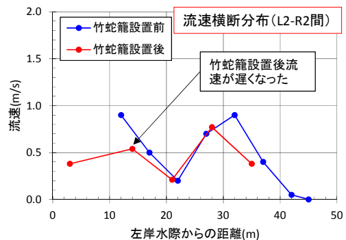
図-16 表面流速 (L2-R2間)
