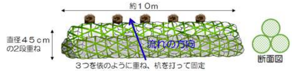
図-4 竹蛇籠のイメージ
