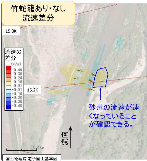
図-9 竹蛇籠あり・なしの河床高差分・流速差分
