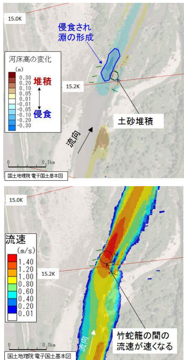
図-7 河床高の変化と流速のコンター図
