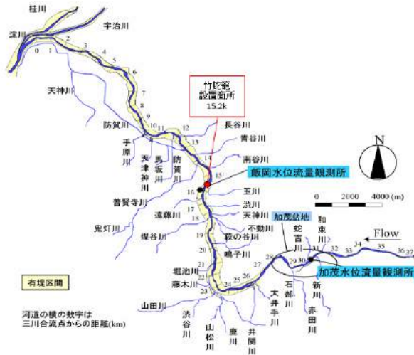
図-1 竹蛇籠設置箇所
