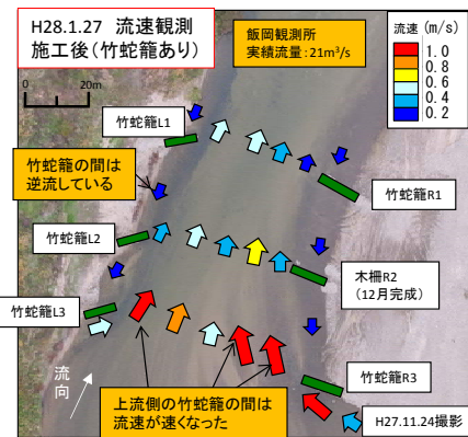
図-14 出水後の表面流速
