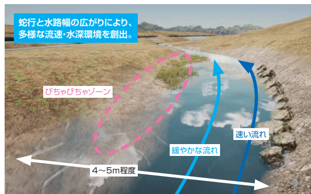
河川環境に配慮した掘削(3次元イメージ図)
