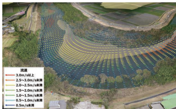
CIMモデル(掘削後の河道と流速計算結果の表示)
